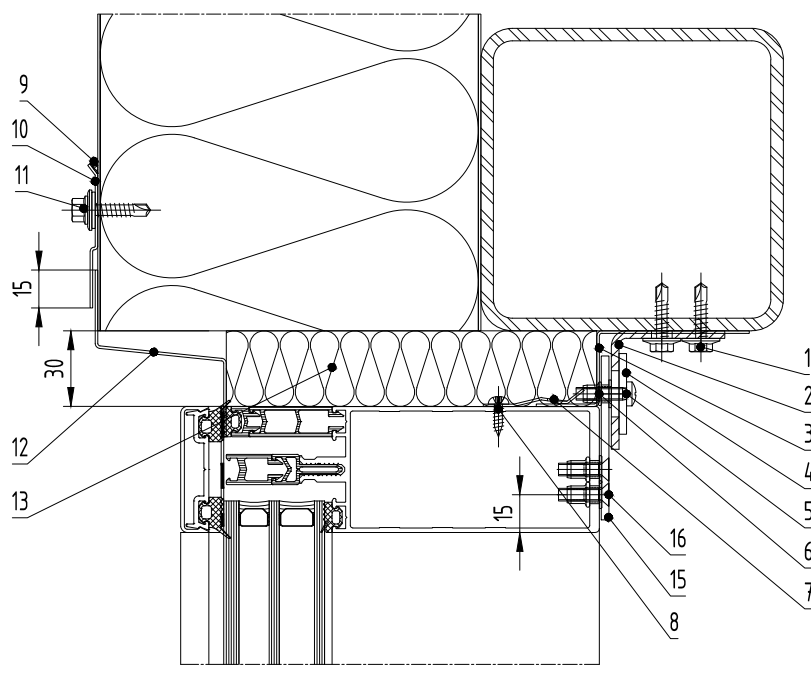
Б-Б
