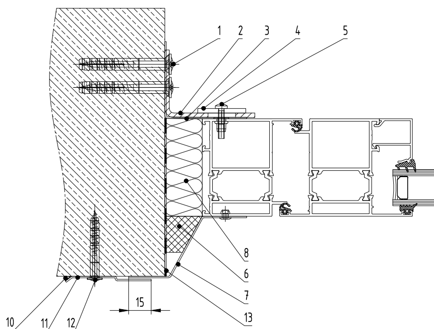
Б-Б
